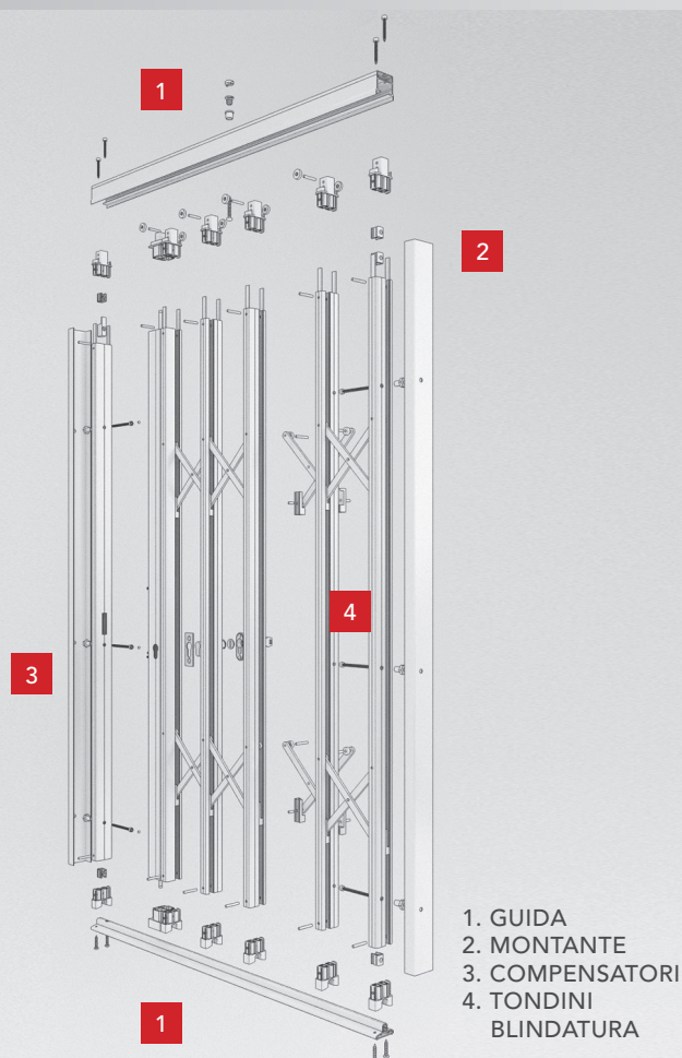
SEZIONE GRATA 2 ANTE
