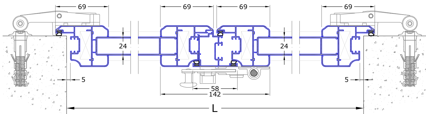
SEZIONE ORIZZONTALE
