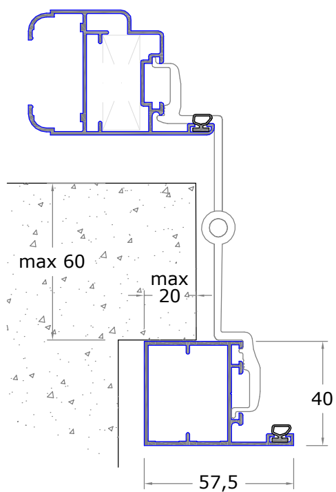
SOLUZIONE CON TELAIO AD ELLE IMPOSTATO DIETRO MAZZETTA
