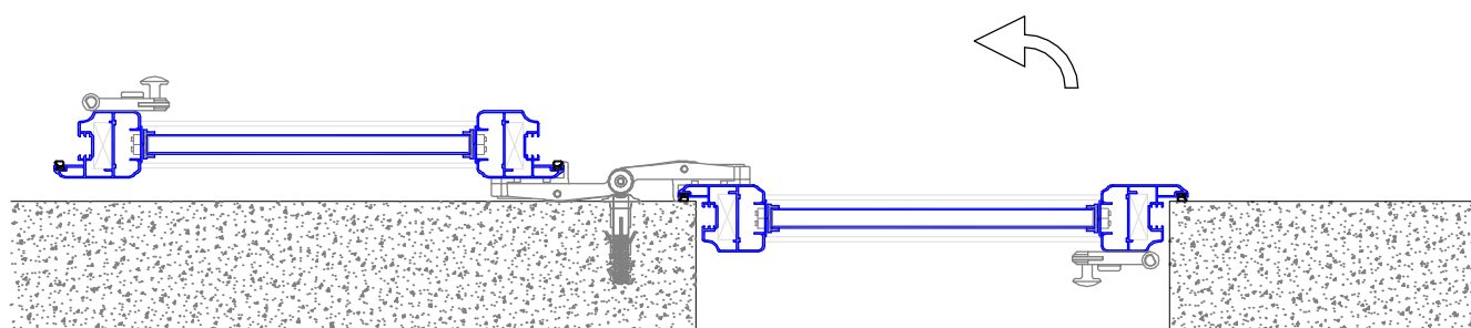
1 ANTA SX - PERSIANA CON CARDINI A MURARE
