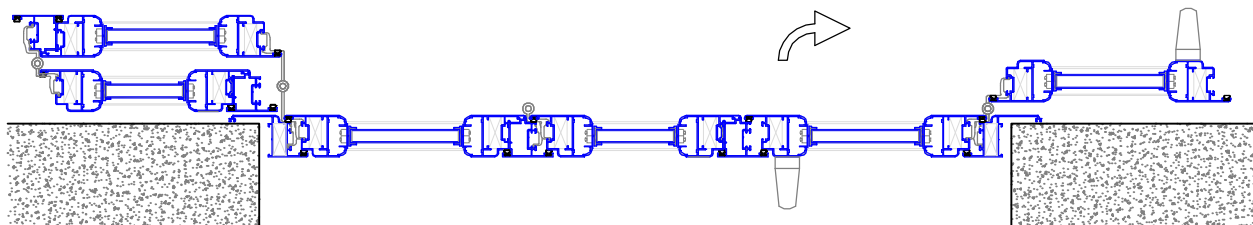
3 ANTE LATERALE DX
