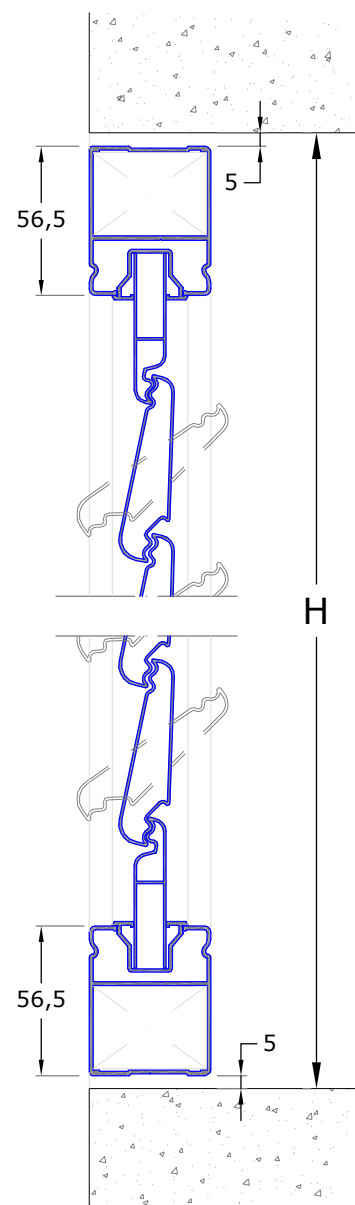
VARIANTE CON BATTUTA 4 LATI
