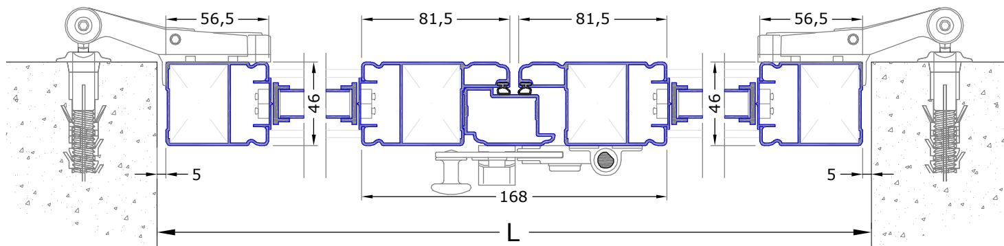
SEZIONE ORIZZONTALE
