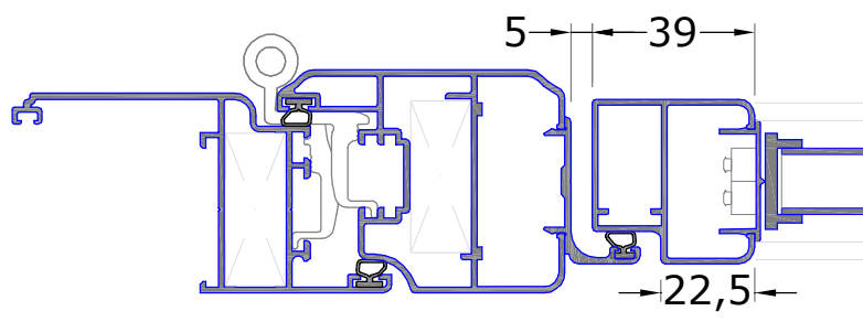
DETTAGLIO NODO LATERALE
