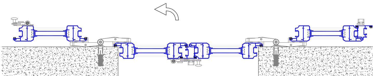
2 ANTE SX - PERSIANA CON CARDINI A MURARE
