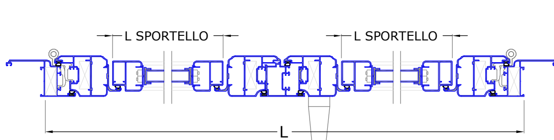
SEZIONE ORIZZONTALE
