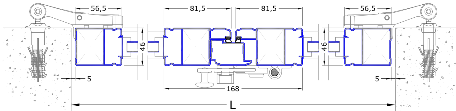
SEZIONE ORIZZONTALE
