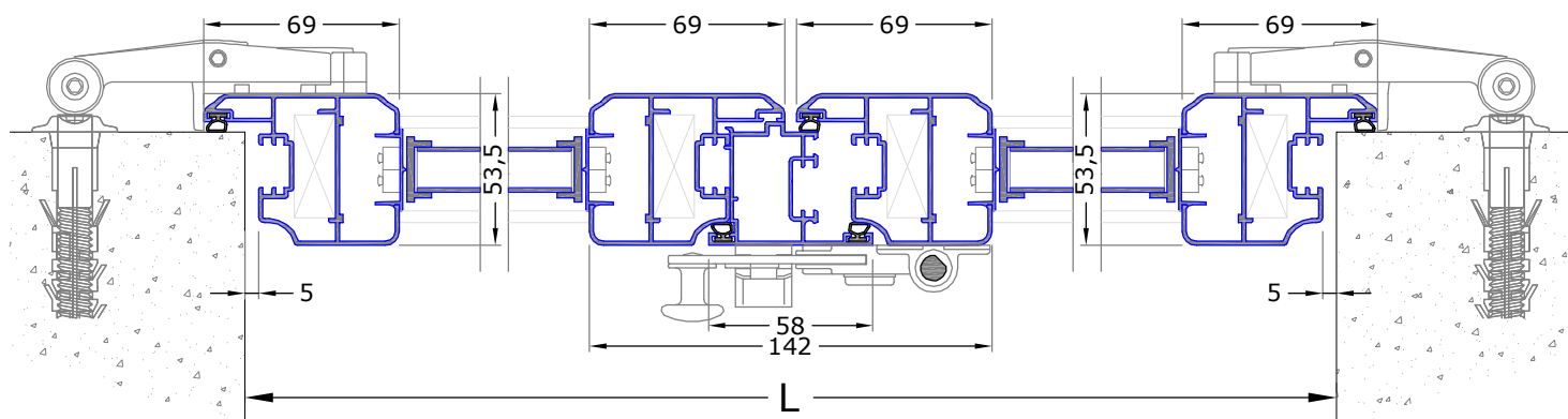
SEZIONE ORIZZONTALE
