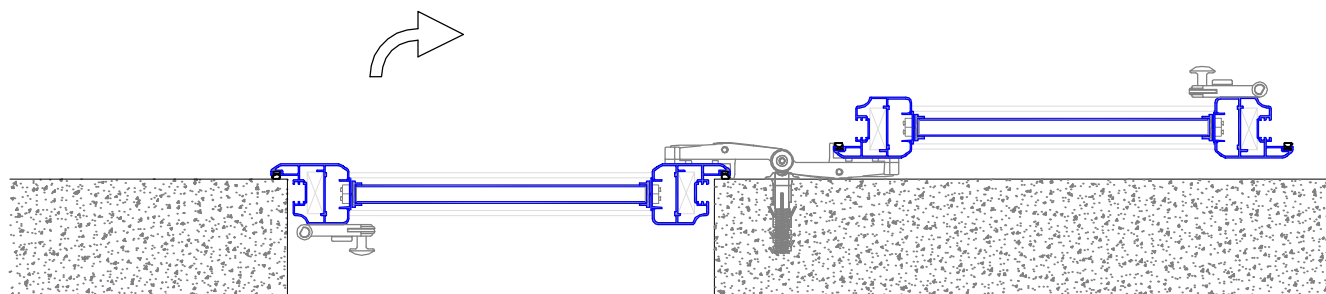
1 ANTA DX - PERSIANA CON CARDINI A MURARE
