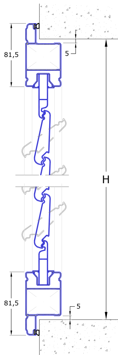
VARIANTE CON BATTUTA 4 LATI
