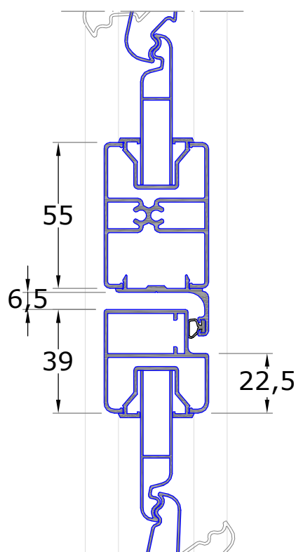
DETTAGLIO NODO VERTICALE
