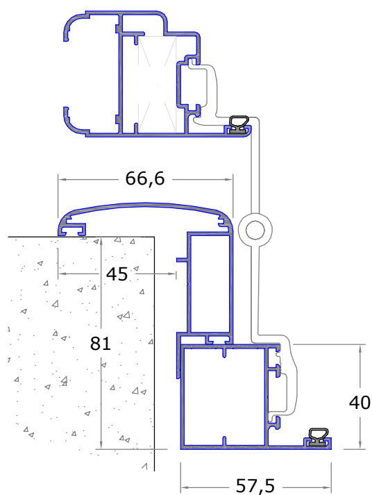
SOLUZIONE CON TELAIO AD ELLE, IMBOTTE E CERNIERE A COLLO ALTO
