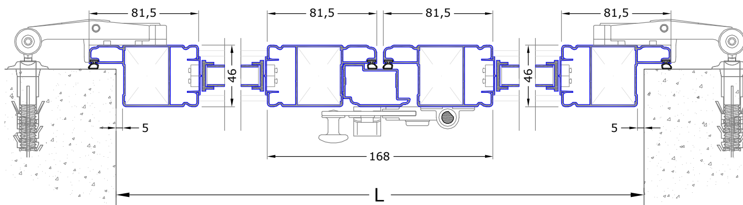
SEZIONE ORIZZONTALE
