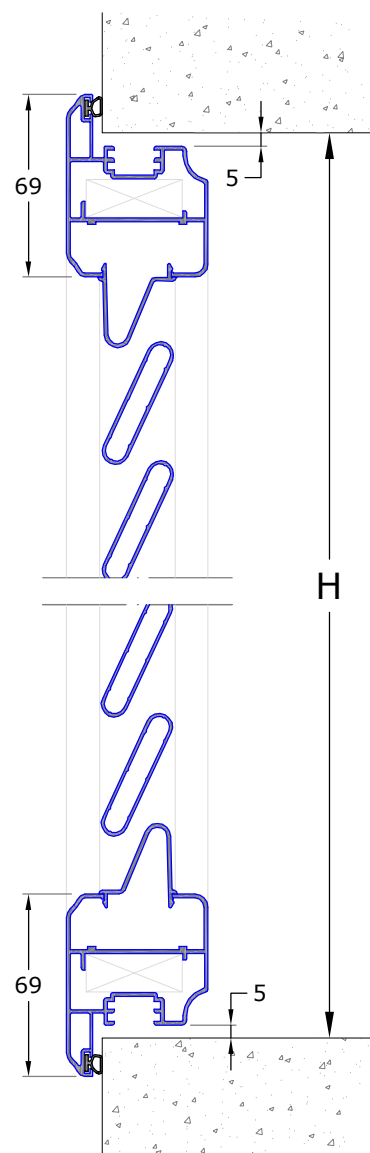
VARIANTE CON BATTUTA 4 LATI
